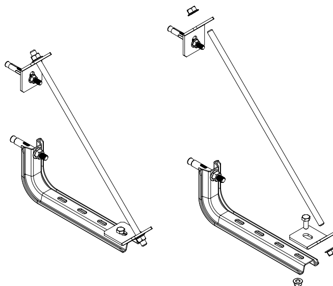
Крепление с СППУ
