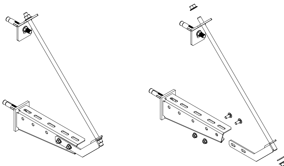
Крепление к стене с одной консолью КПН5
