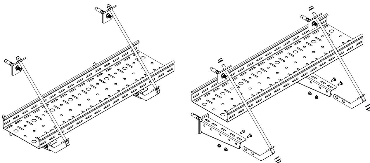
Крепление к стене с ПНУ
