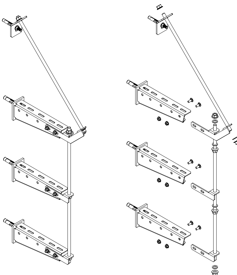
Крепление к стене с тремя консолями КПН5
